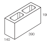
15.01 Standard Block/ Double Corner 12.8kg 95 per pallet
