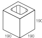
20.03 Half 9.0kg 150 per pallet
