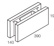
15.91 Double 'U' Block 13.1kg 95 per pallet
