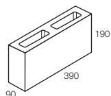
10.01 Partition 11.2kg 158 per pallet
