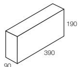
10.31 Solid Partition 14.3kg 126 per pallet
