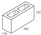
15.201SB Double Corner 12.8kg 95 per pallet
