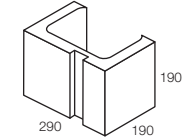
30.15 Half End 12.5kg 125 per pallet
