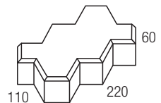
Interpave 60®
