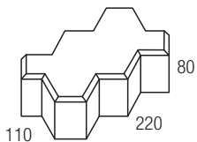
Interpave 80®
